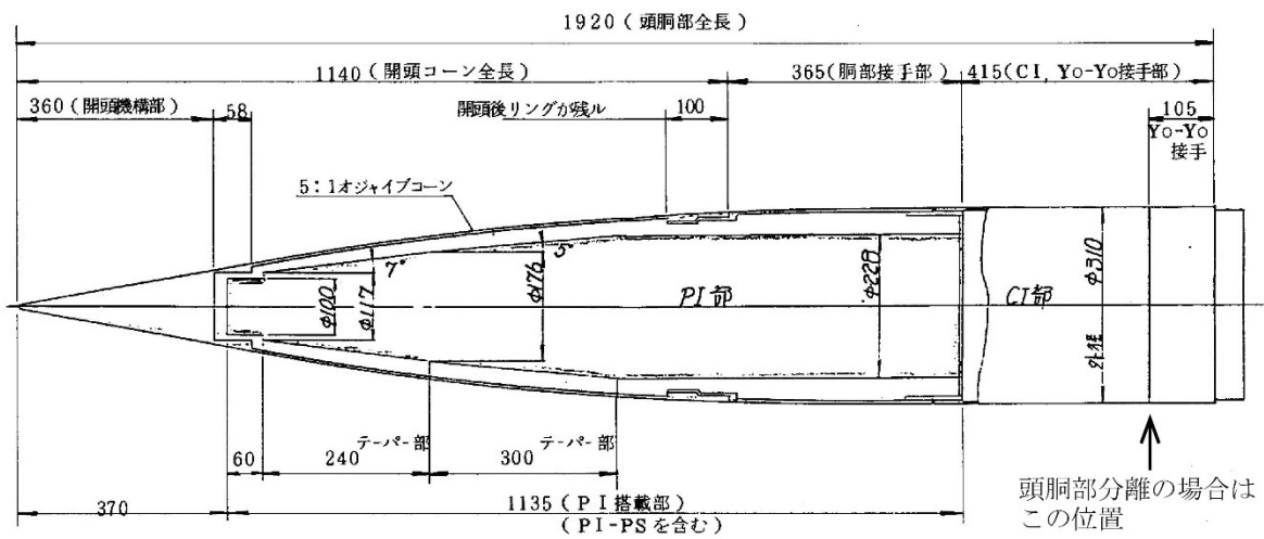
S-310 標準型観測機器搭載部寸法図
