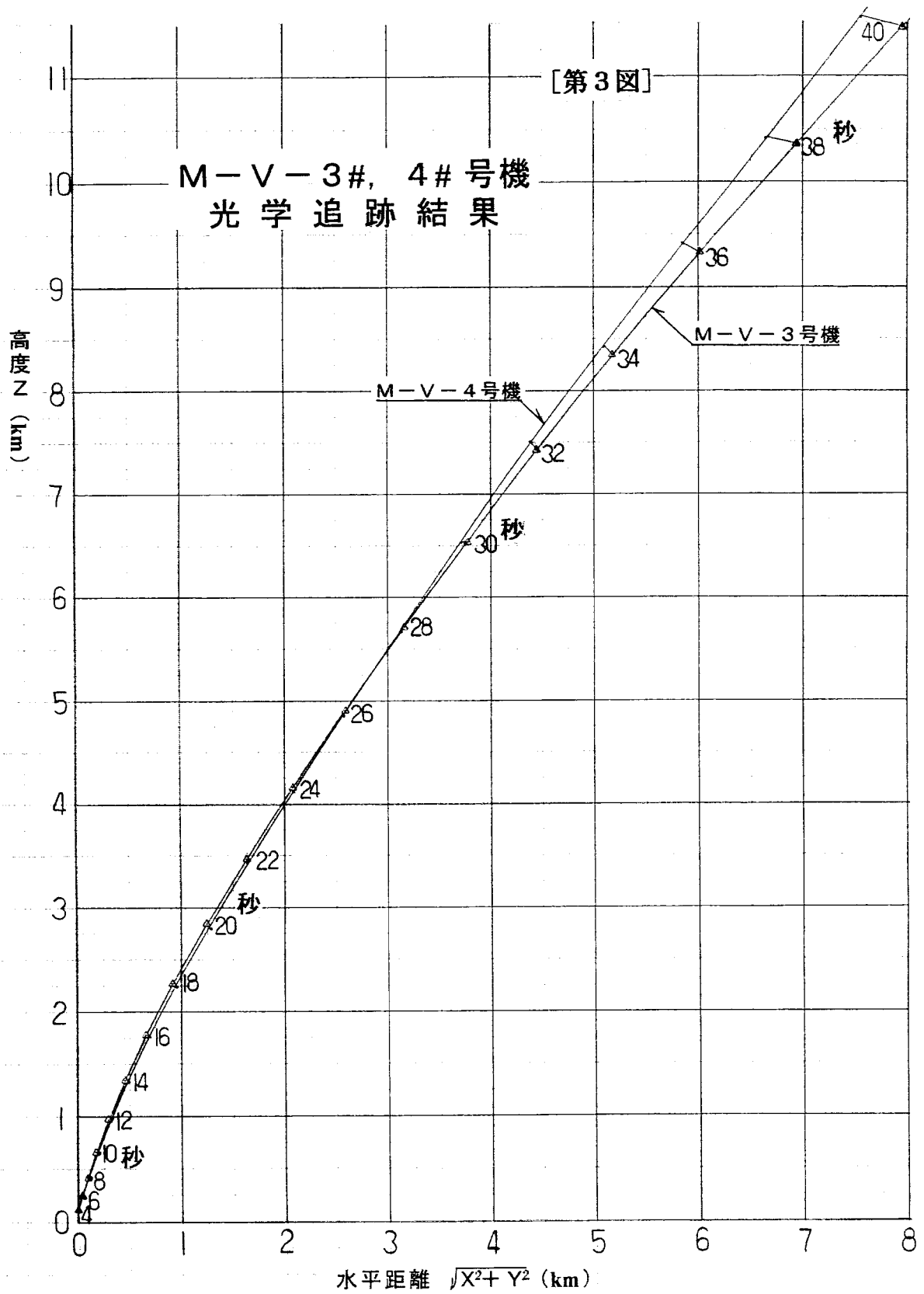
図3 M-V-3, 4号機 光学追跡結果
