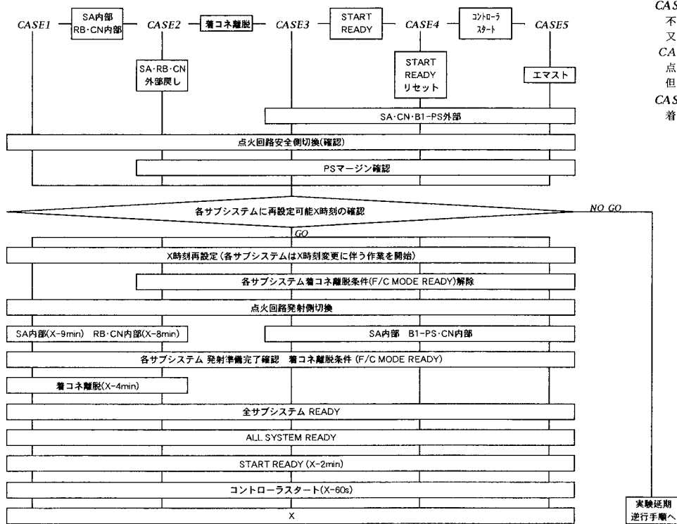
図1.4 M-V-4 号機 X時刻変更手順
