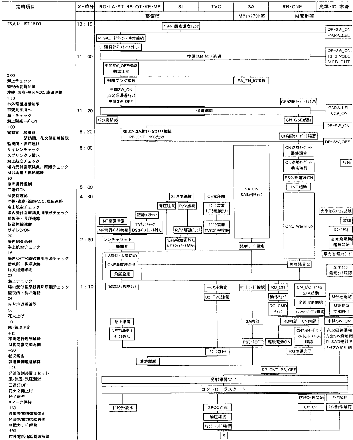
図1.2 M-V-3号機タイムスケジュール
