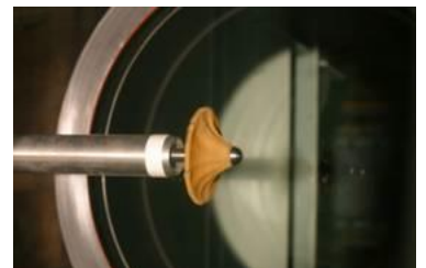
はやぶさカプセル・柔軟構造エアロシェルの試験用模型
