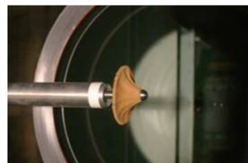
はやぶさカプセル・柔軟構造エアロゲルの試験用模型
