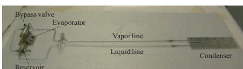
〈ループヒートパイプ〉
