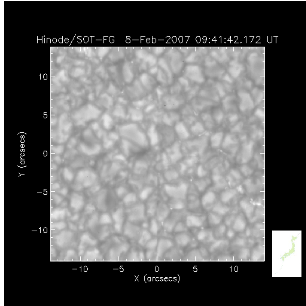
えいせい かしこうじばほうえんきょう たいようひょうめん ひので衛星可視光磁場望遠鏡でみた太陽表面
