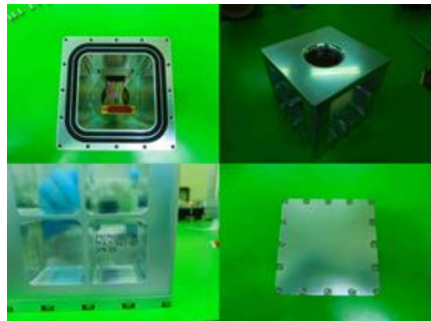
図3 2020 年度に作製した与圧部モジュール試作 1号機の外観
