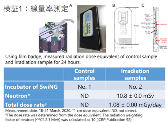
Fig. 3. SwiNG の線量率測定結果
