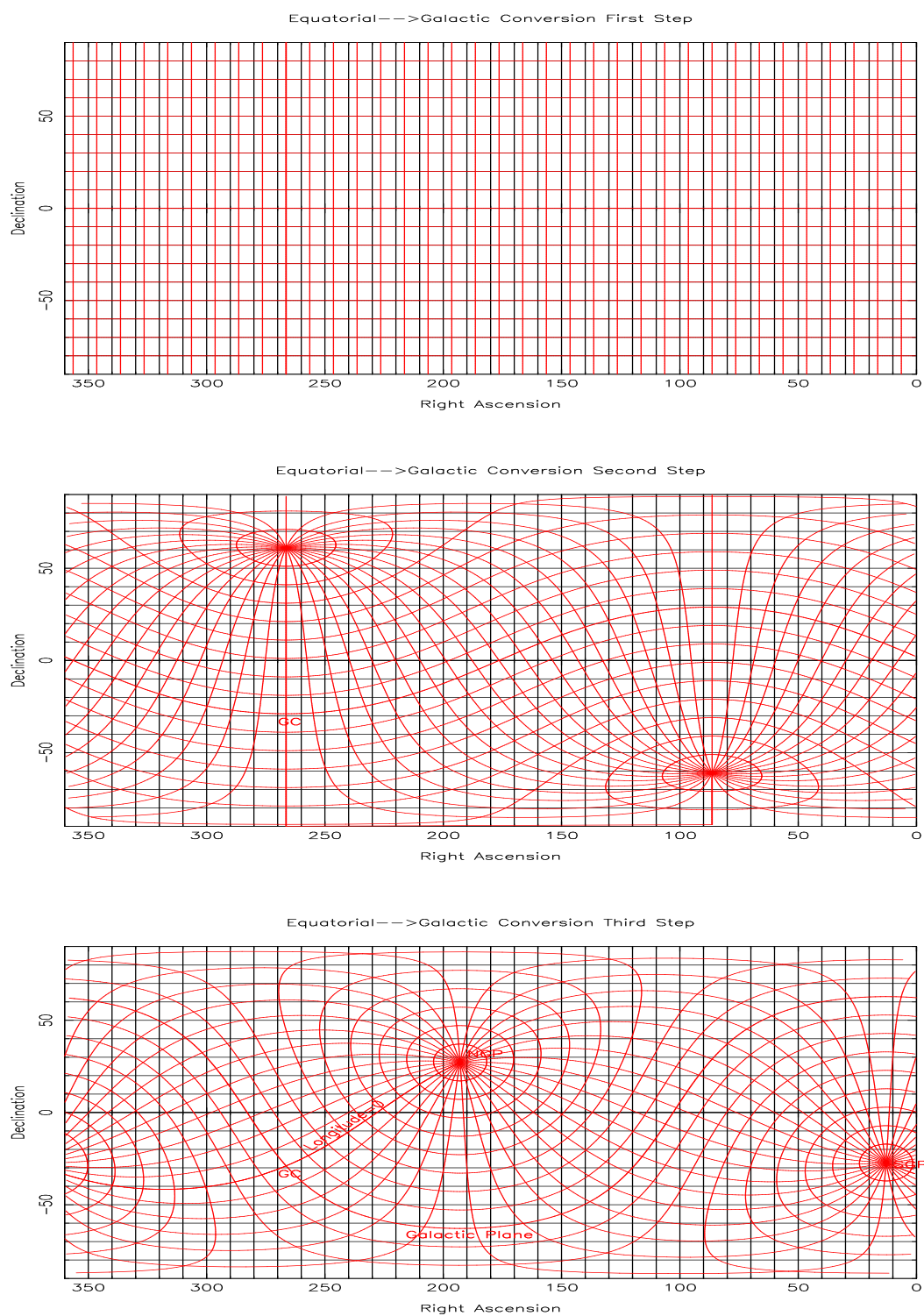
Figure 2: 赤道座標から銀河座標への変換
