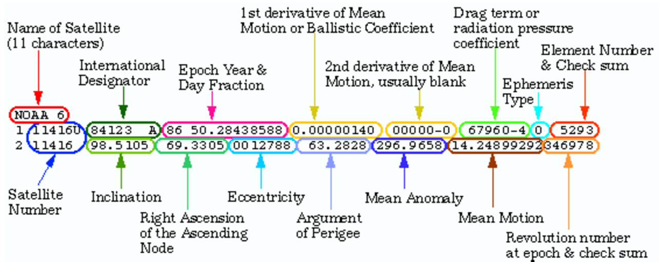
Fig. 10. 人工衛星の軌道と位置を記述する Two Line Elements (TLE) の説明。 http://science.nasa.gov/Realtime/rocket_sci/orbmech/state/2line.html より。
