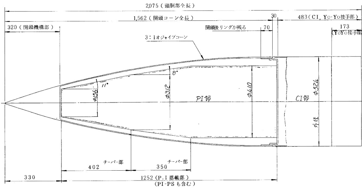
S-520、SS-520 標準型 観測機器搭載部寸法図
