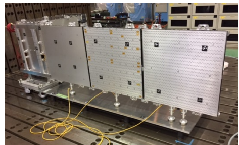
アンテナパネル展開完了状態(片翼)
